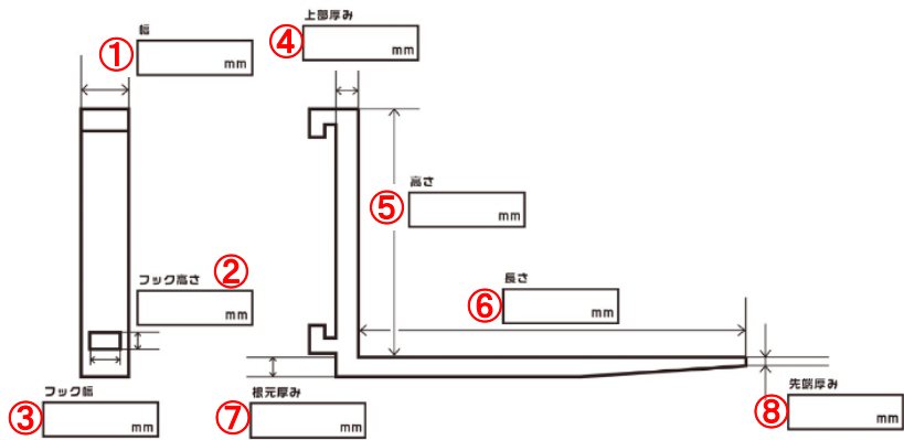
ツメ寸法図
